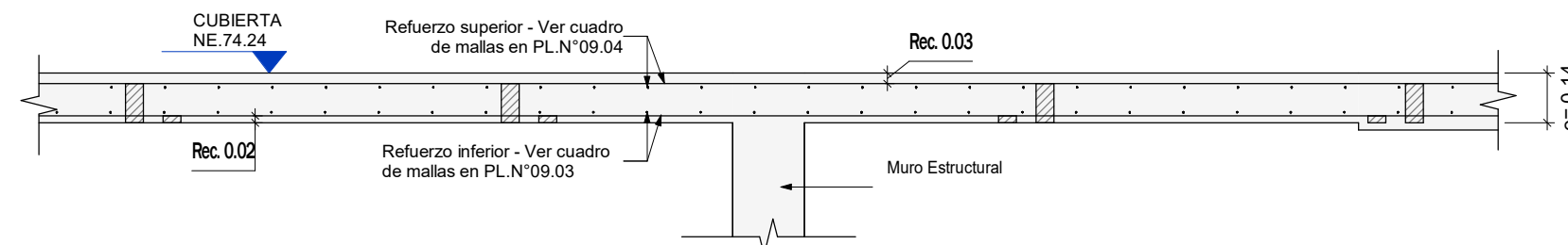
CORTE TÍPICO PLACA AÉREA e=0.14 Escala 1 : 20
