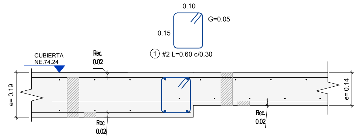
DETALLES TÍPICOS - CAMBIO DE SECCIÓN Escala 1 : 10
