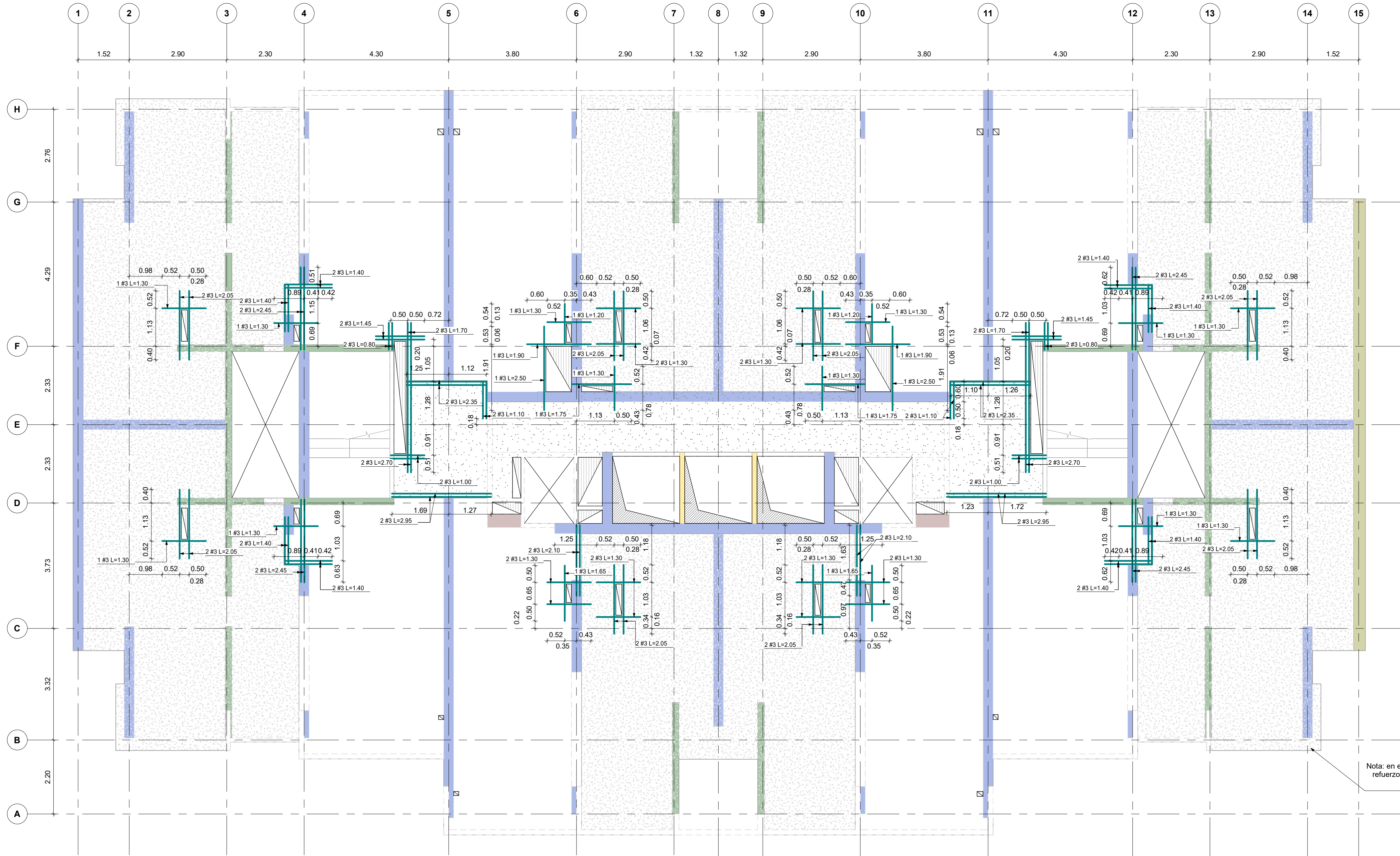
PLANTA DE REFUERZO ADICIONAL (INFERIOR Y SUPERIOR) CUBIERTA Escala 1 : 75
