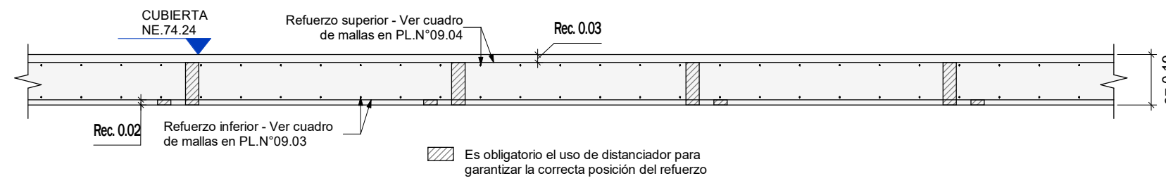
CORTE TÍPICO PLACA AÉREA e=0.19 Escala 1 : 20
