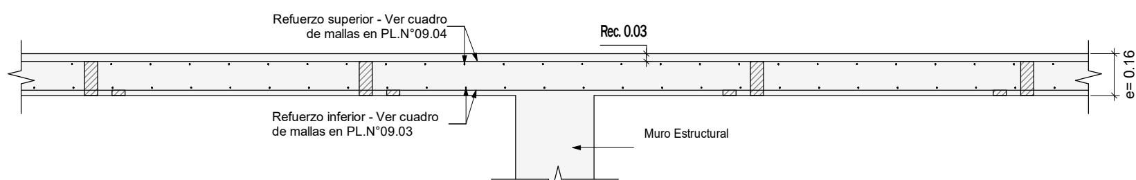
CORTE TÍPICO PLACA AÉREA e=0.16 Escala 1 : 20
